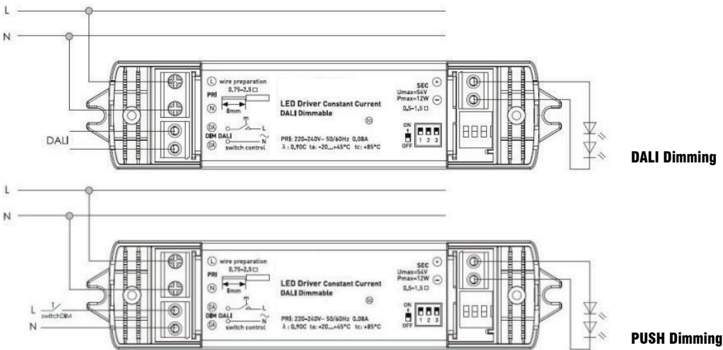
Wiring diagram - Schema di collegamento
