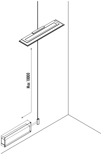
KIT DI ALIMENTAZIONE REMOTO / REMOTE POWER SUPPLY KIT
