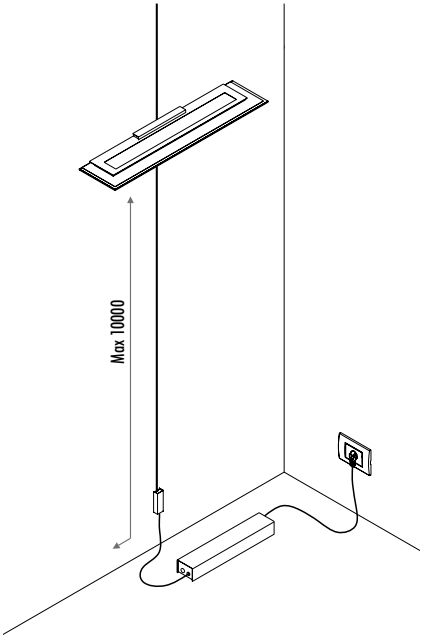
KIT DI ALIMENTAZIONE CON SPINA / POWER SUPPLY KIT WITH PLUG
