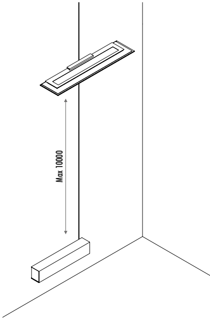
KIT ROSONE DA PARETE E SOFFITTO / WALL AND CEILING ROSE KIT
