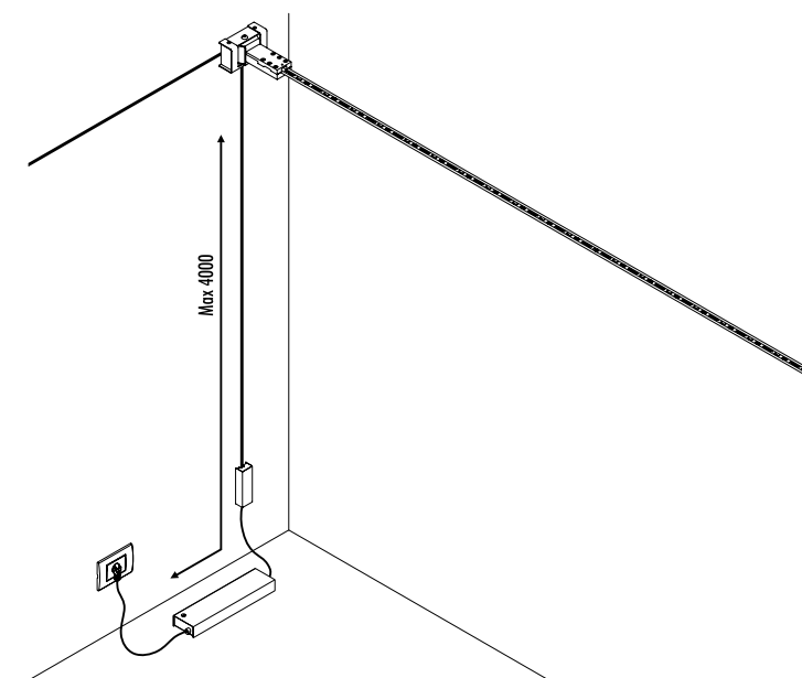
INSTALLAZIONE CON ENDLESS E KIT DI ALIMENTAZIONE CON SPINA / INSTALLATION WITH ENDLESS AND POWER SUPPLY KIT WITH PLUG
