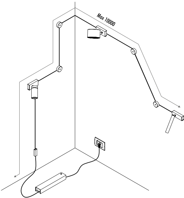
KIT ROSONE DA PARETE E SOFFITTO / WALL AND CEILING ROSE KIT
