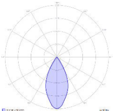
BB-TUBE 60°
