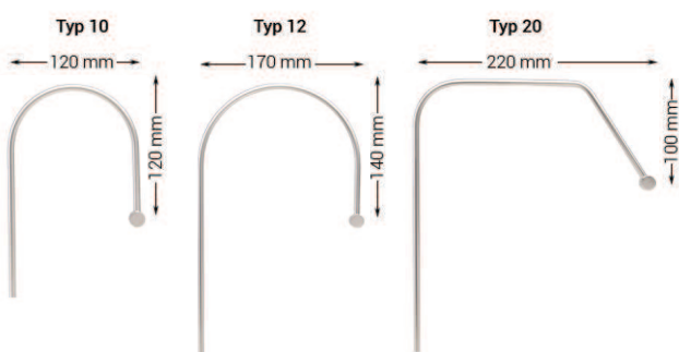
Bügeltypen:
