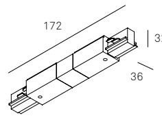
MLN Guia / 8502 AL L. 172 Max. 3600 W.
