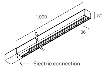
MLN Guia / 8500 AL L. 1000 Max. 3600 W.
