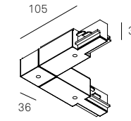
MLN Central Connector / 8503 interior / 3503 exterior AL L. 105 | Max. 3600 W.
