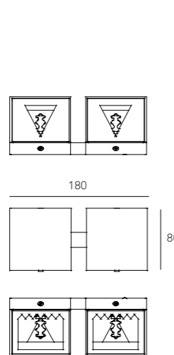
MLN Dau / 6022 Flemming Bjorn AL Ø 180 | H 80 | S 101 2 x G9 | 42 W. Eco ⊕ | ▽ | ◡ Dim. | EEI: D
