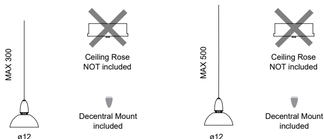
Galileo Mini LED M
