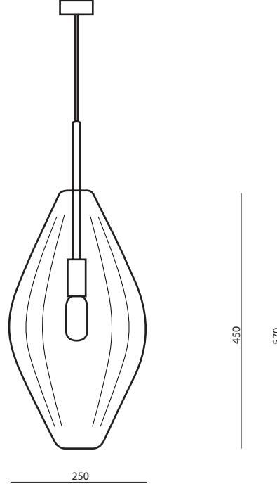
Bailey pendant
